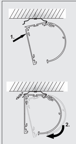
Plafond montage
